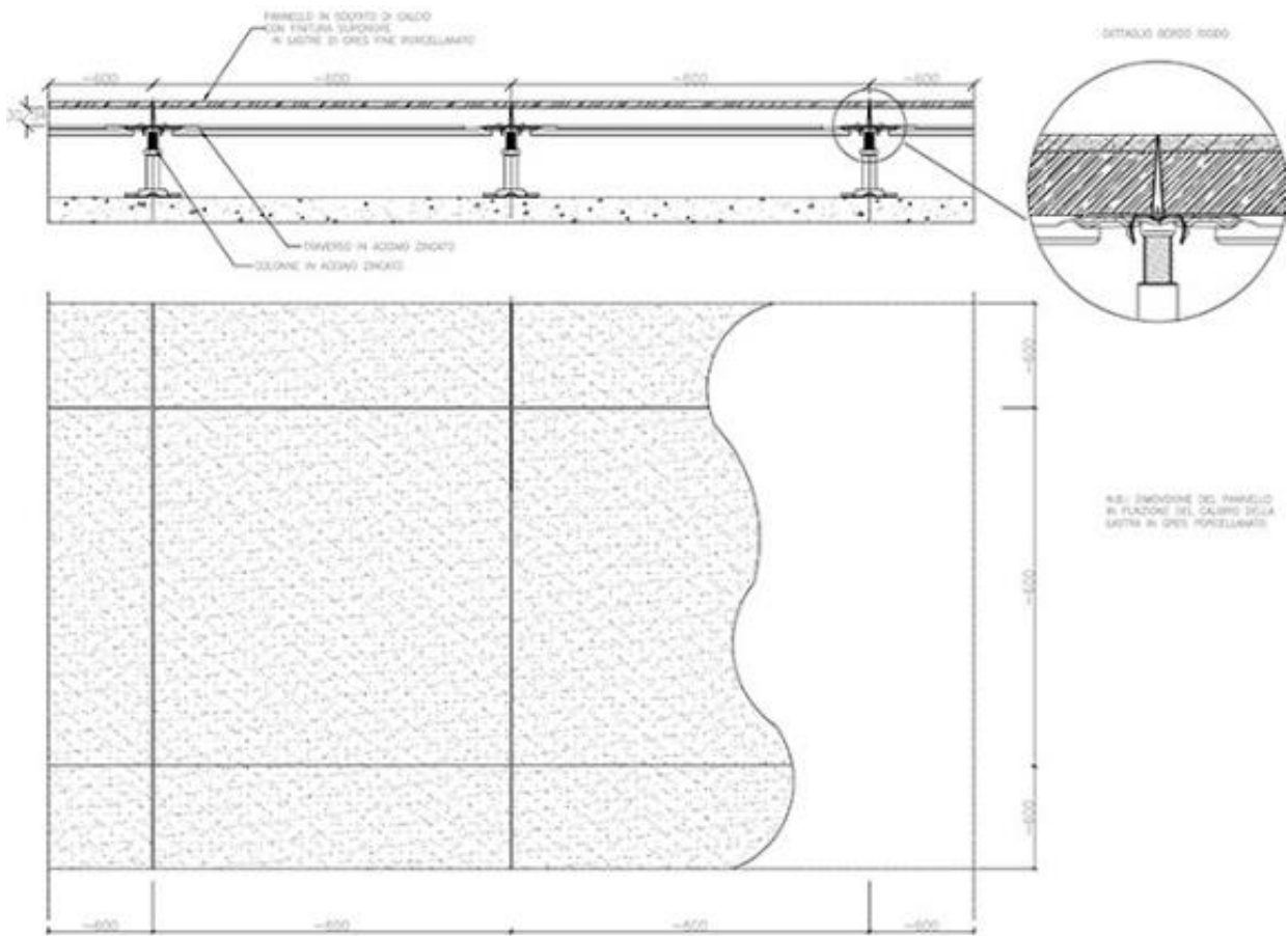
SEZIONE
